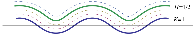
図 1: unduloid (平均曲率一定回転面) とその平行曲面族の母線
