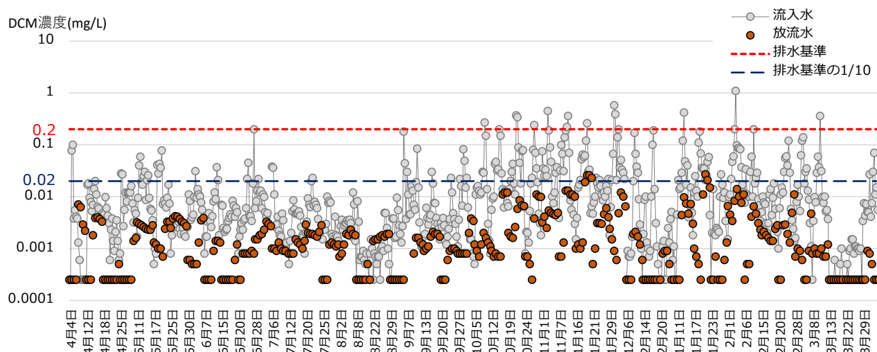
図 5.1.9 2022 年度の 5 号館排水処理施設流入水及び放流水のジクロロメタン (DCM) 濃度 流入水と放流水のジクロロメタン濃度の変動の様子を対数表示したもの。
