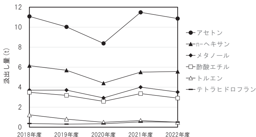
図 5.1.11 溶媒の年間汲出し量の経年変化（2018～2022 年度）
