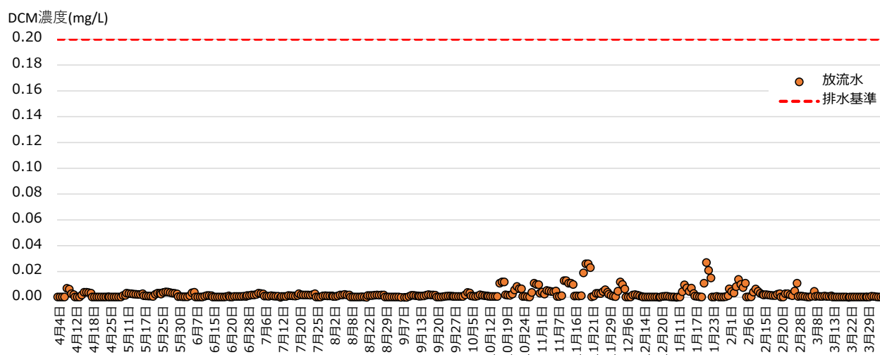
図 5.1.8 2022 年度の 5 号館排水処理施設の放流水中ジクロロメタン (DCM) 濃度 放流水（排水基準適用対象）のジクロロメタン濃度の変動の様子（毎週の測定日の 2 時間ごとの測定結果）を連続的に示す。
