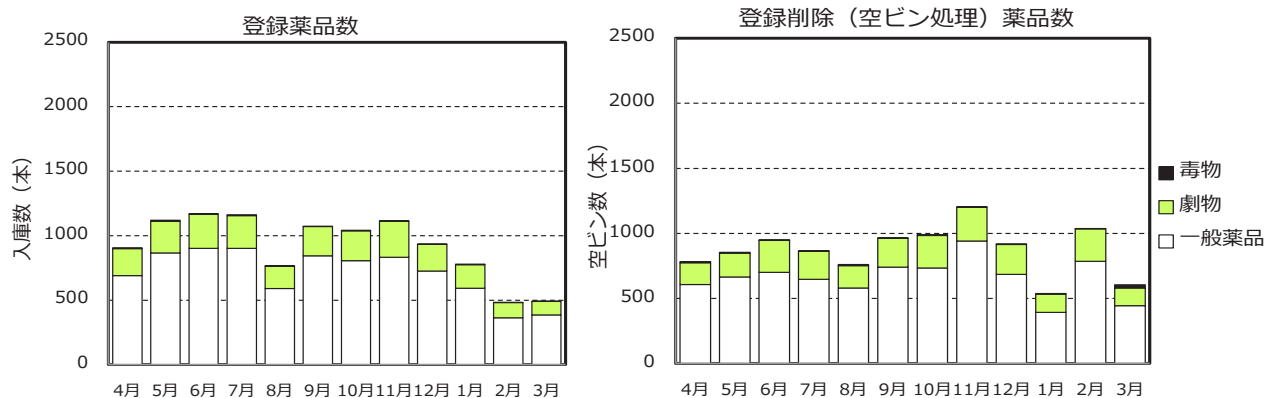
図 5.1.3 神楽坂キャンパスの薬品管理状況（2022 年度）
