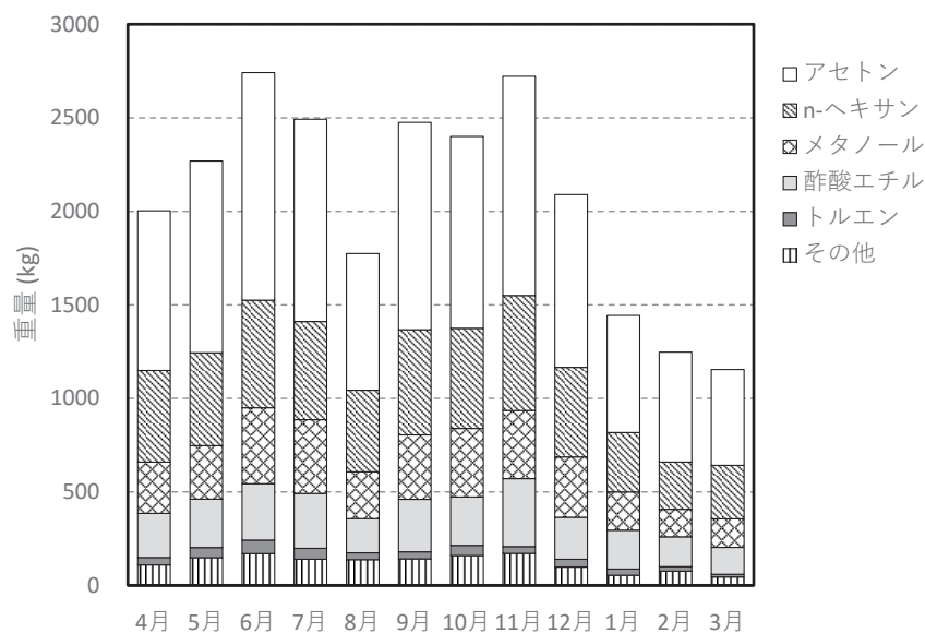
図 5.1.12 の 1 溶媒の汲出し量の月変化（2022 年度）
