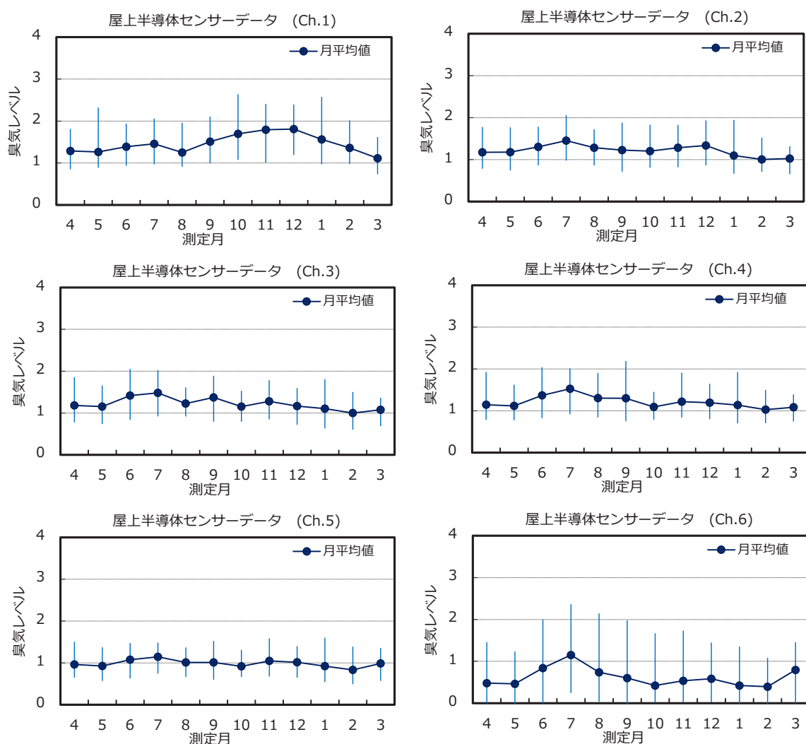
図 5.1.10 神楽坂キャンパス 5 号館屋上における揮発性物質の常時監視結果 (2022 年度)
