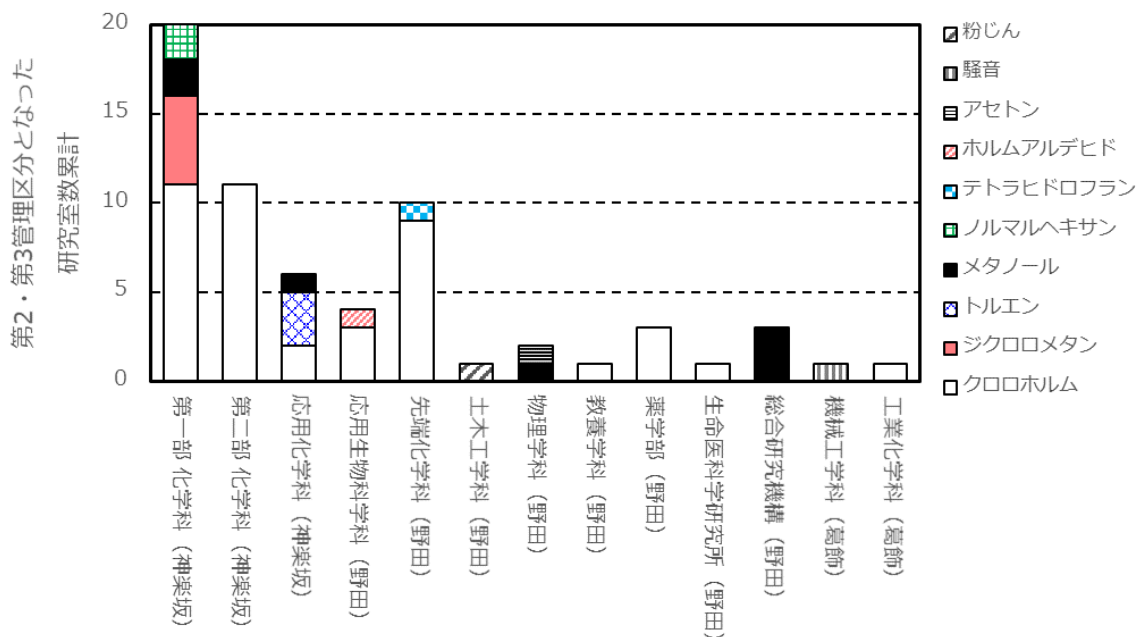
図 5.2.1 第 2・第 3 管理区分の原因となった物質 (2018～2022 年度)
