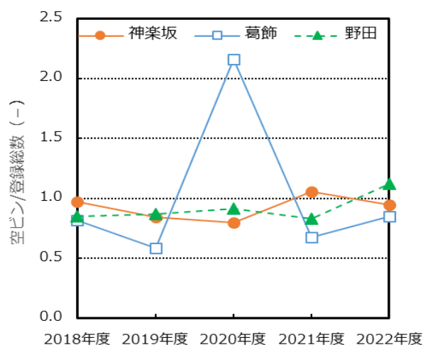
図5.1.2 入出庫登録比率の経年変化(2018-2022年)
