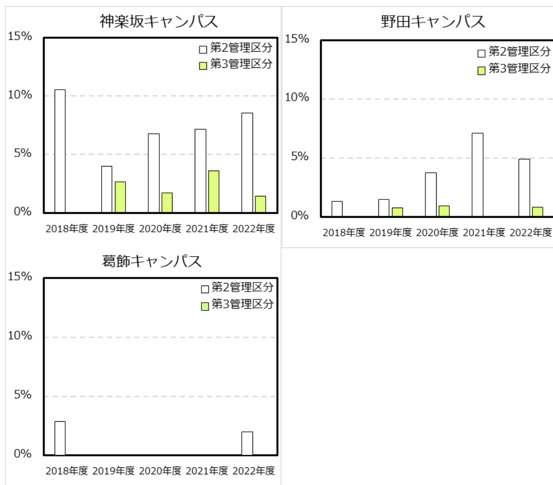
図 5.2.2 各キャンパスの第2・第3管理区分比率の推移（2018～2022年度）
