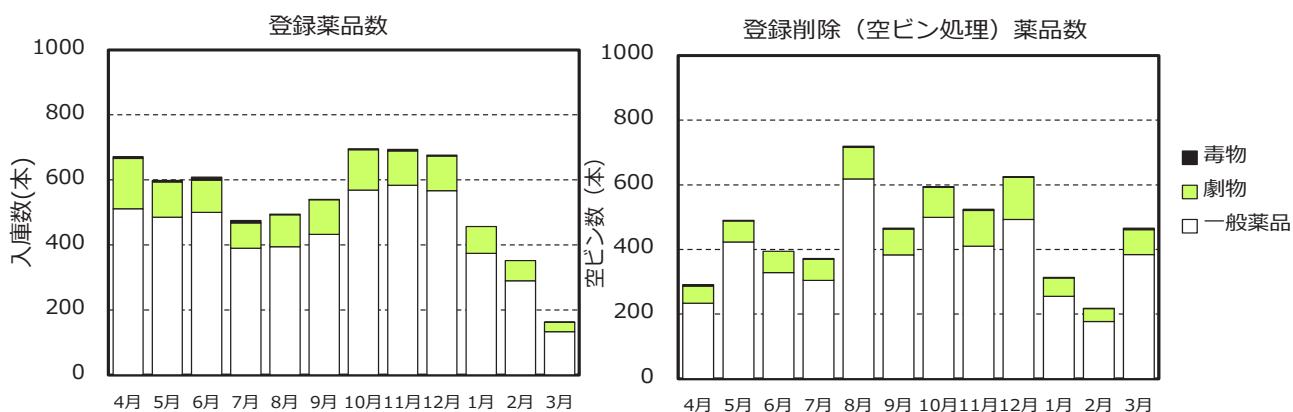
図 5.1.5 葛飾キャンパスの薬品管理状況（2022 年度）
