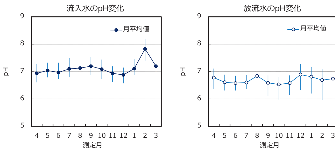
図 5.1.6 神楽坂キャンパス 5 号館の流入水と放流水の水素イオン濃度 (pH) の月別推移 (2022 年度)
