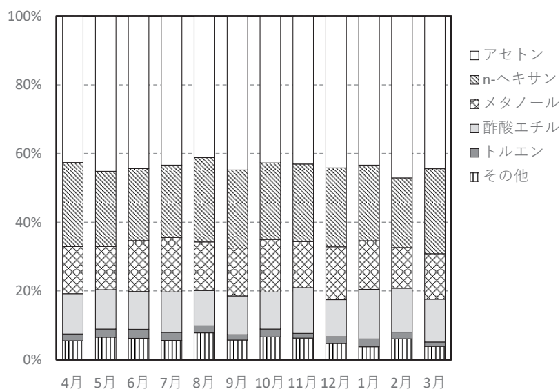
図 5.1.12 の 2 溶媒の汲出し比率の月変化（2022 年度）
