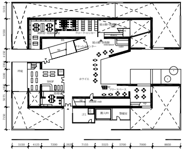
一階平面図 1:1200
