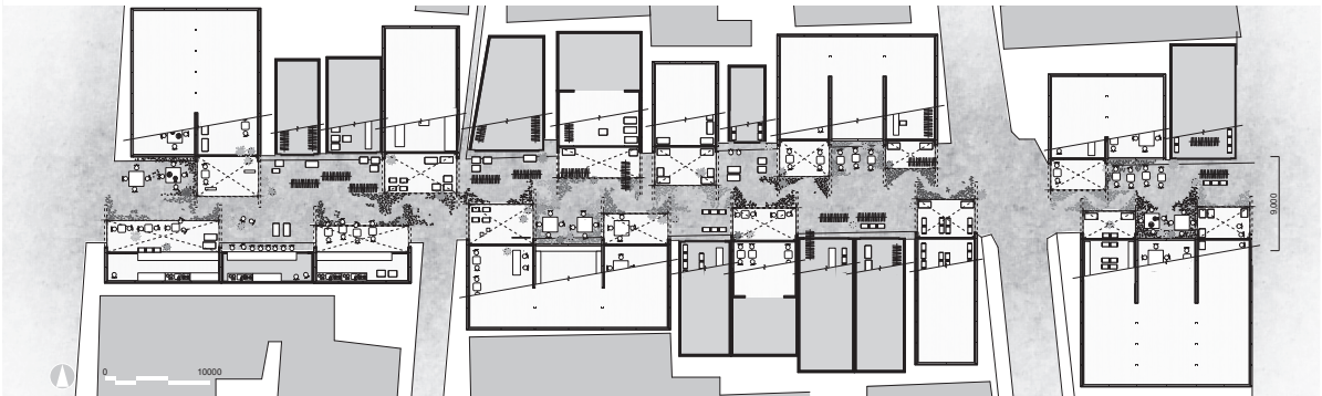
-site plan 1/800
